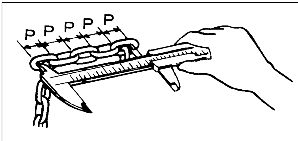
Kuva 5 Kuormaketjun kontrollimittaus
